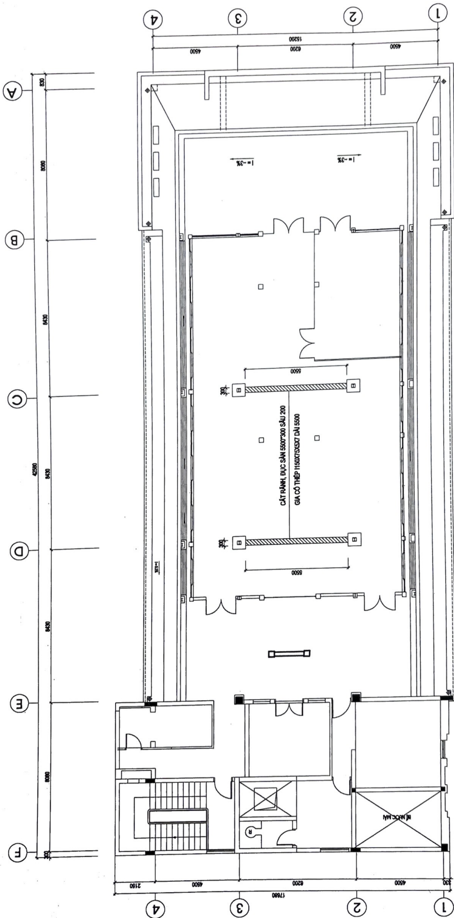
MẶT BẰNG GIA CỐ KẾT CẤU SÀN
