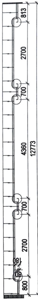
MẶT CẮT A-A - TRẦN THẠCH CAO - PHÒNG ẨM VIP
