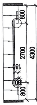
MẶT CẮT B-B - TRẦN THẠCH CAO - PHÒNG ẨM VIP
