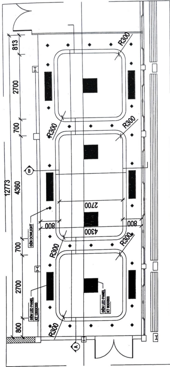
MẶT BẰNG - TRẦN THẠCH CAO - PHÒNG ẨM VIP
