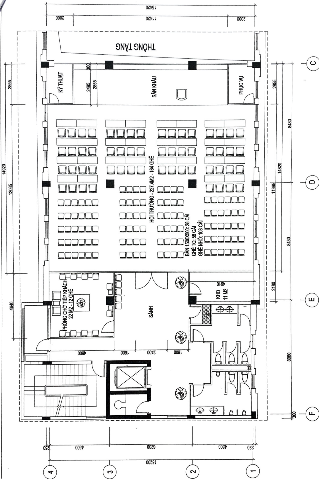
MẶT BẰNG CẢI TẠO TẦNG M2 (DỰ KIẾN) - TÒA NHÀ 81 TRẦN HƯNG ĐẠO
